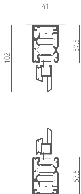
iestiklojuma sistēma glazing system
