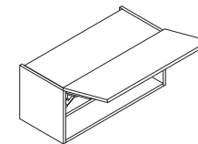
paceļamas durvis, 1 plaukts W 600-1000, H 360, D 360 flap opening, 1 shelf W 600-1000, H 360, D 360
